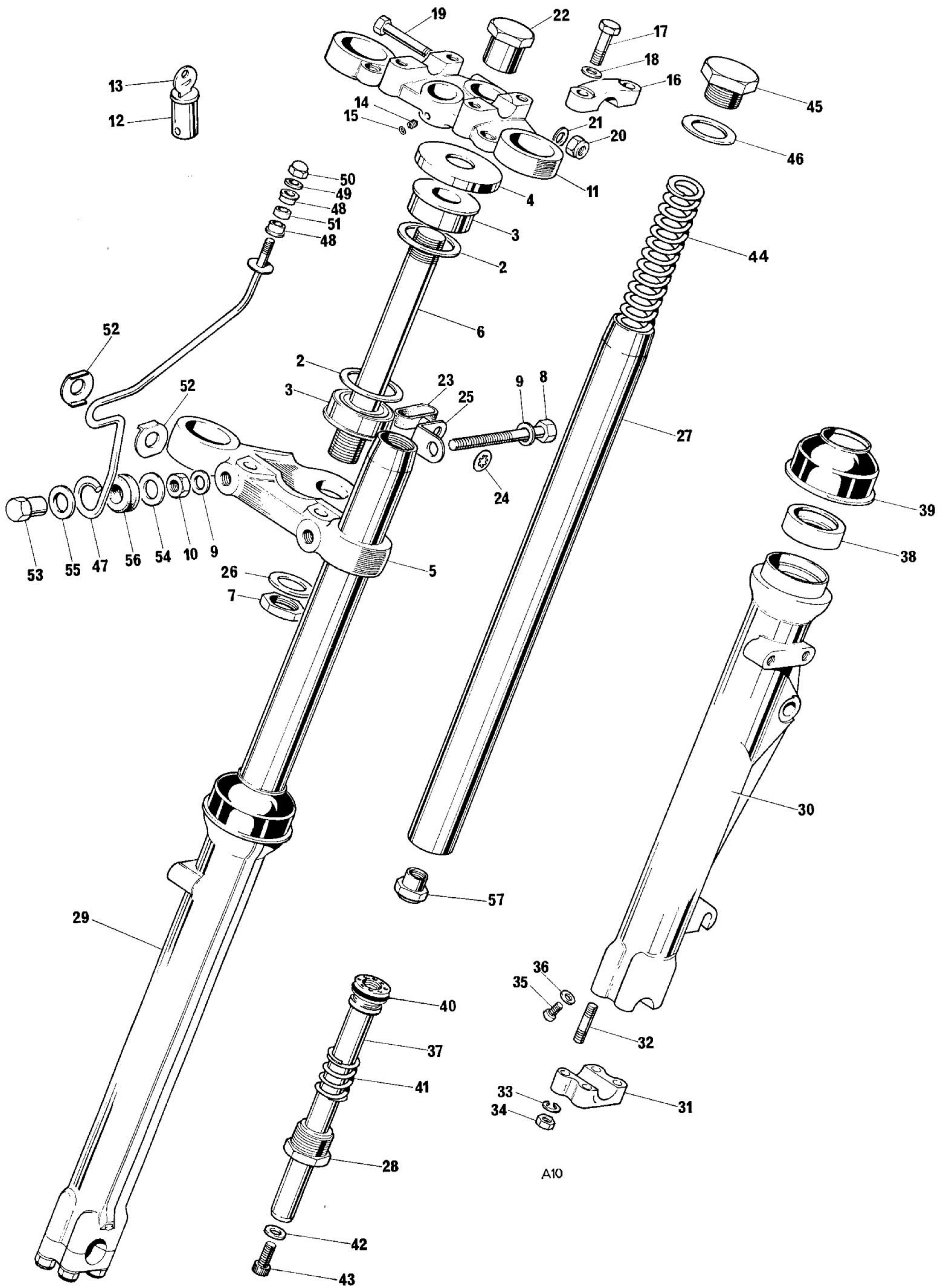
Fig. 10. TELESCOPIC FORKS
