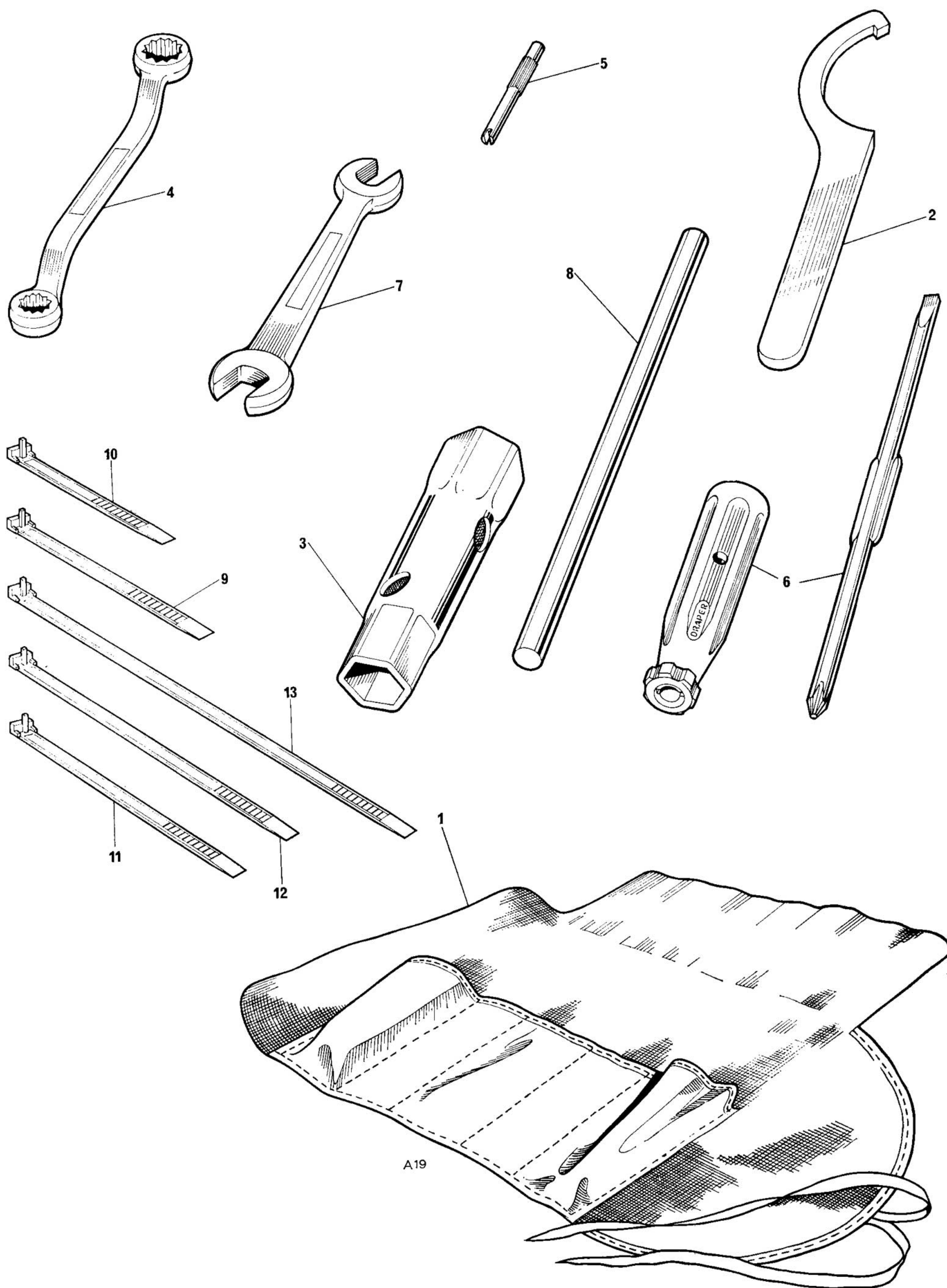
Fig. 19. TOOL KIT
