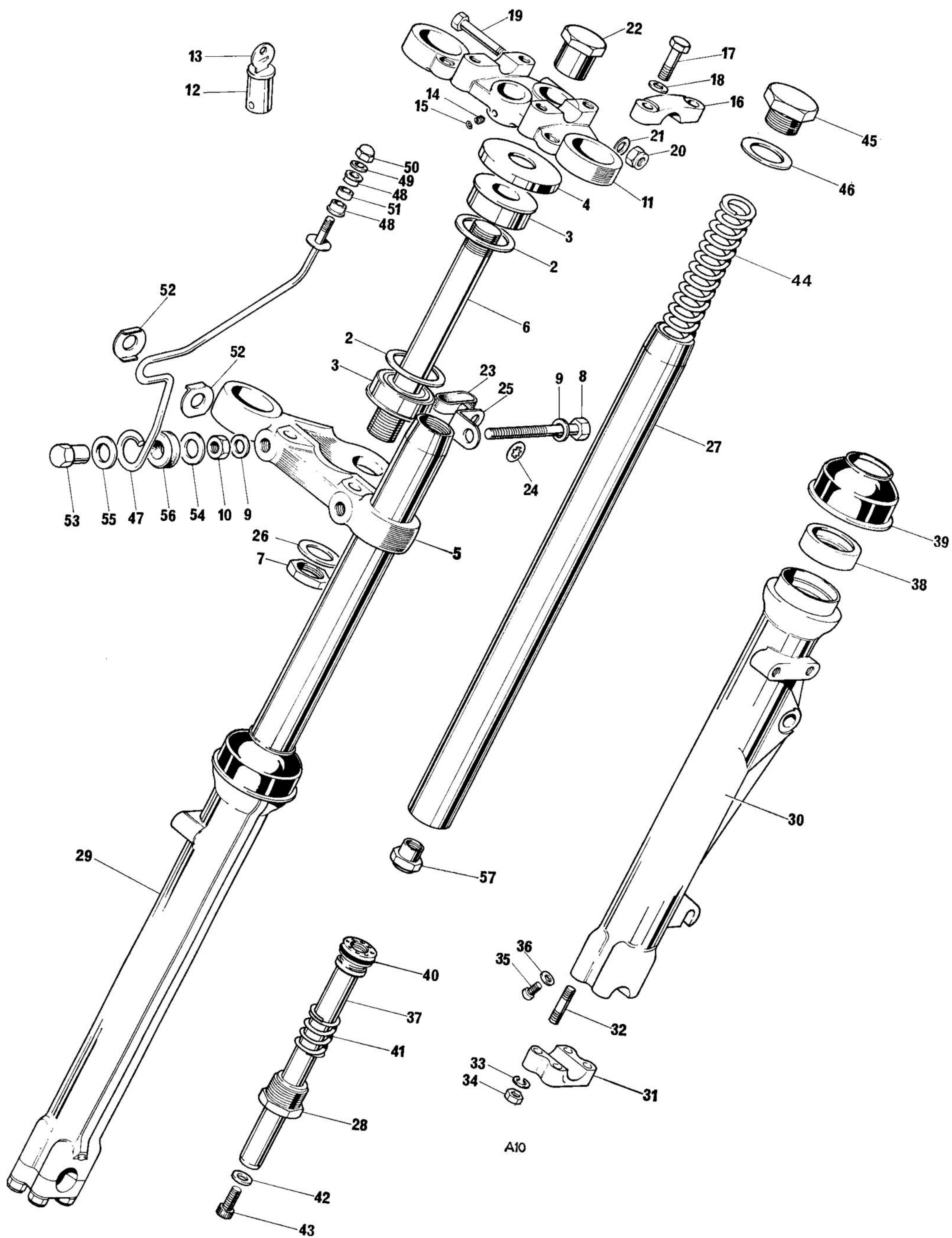
Fig. 10. TELESCOPIC FORKS
