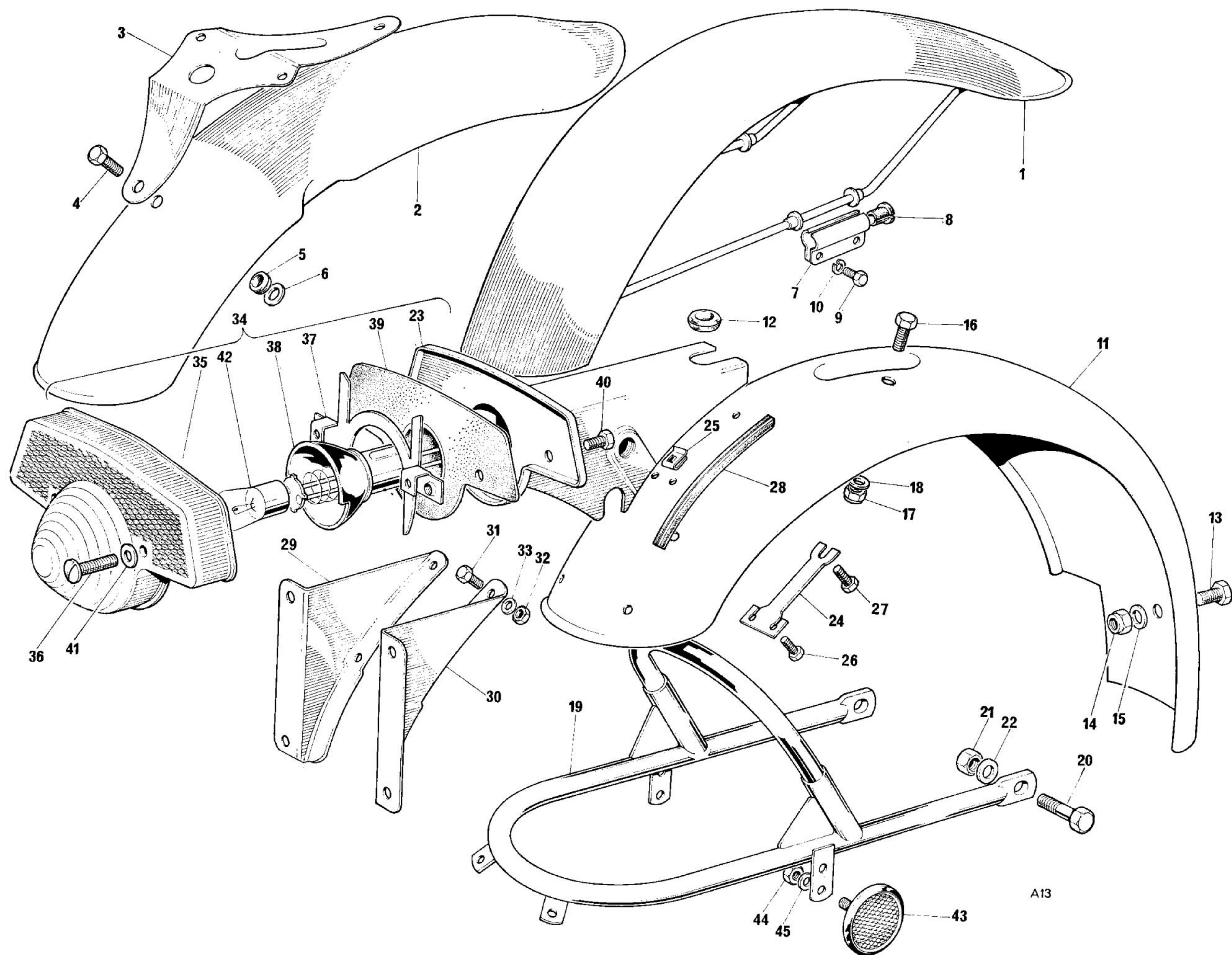
Fig. 13. FENDERS
