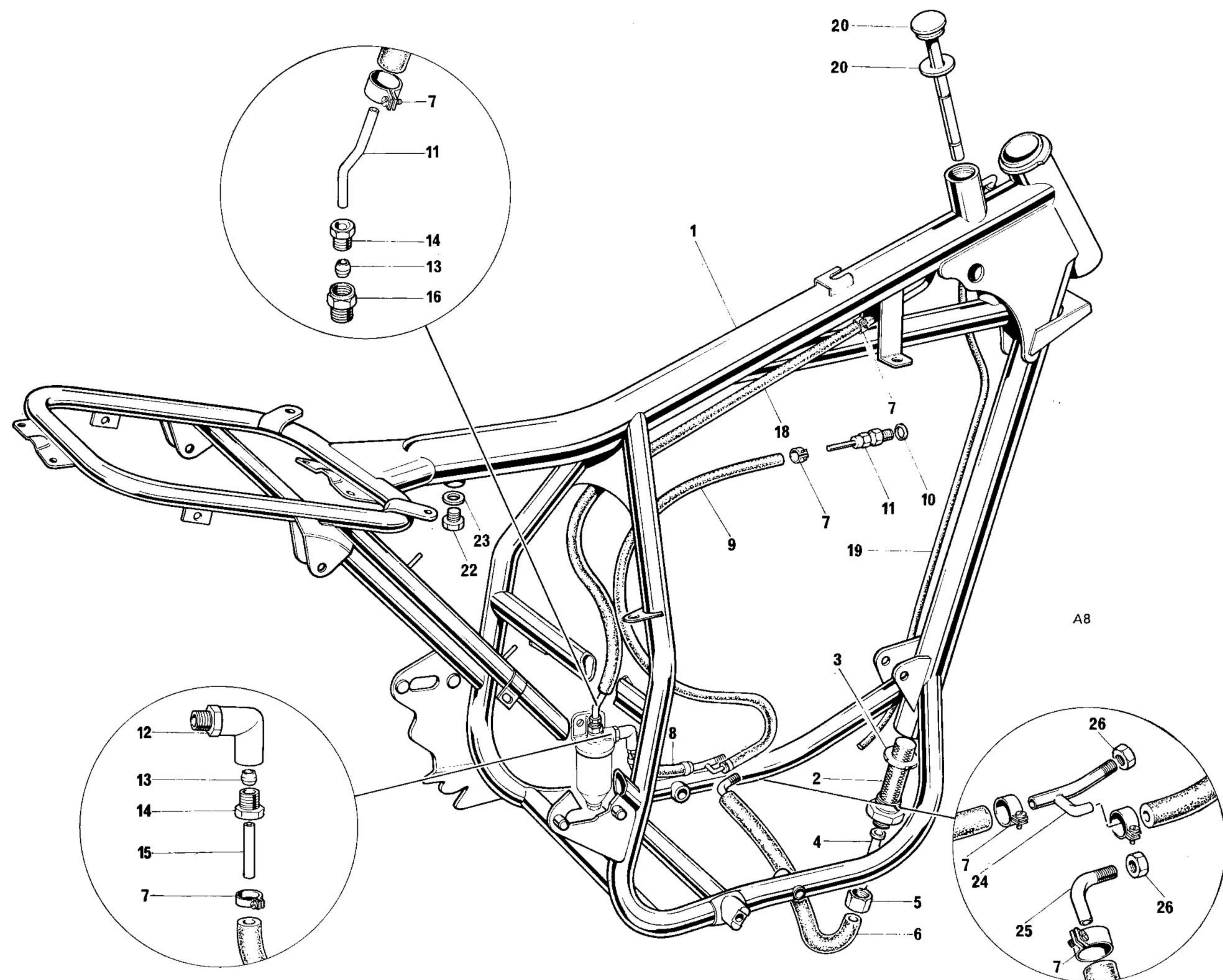
Fig. 8. FRAME
