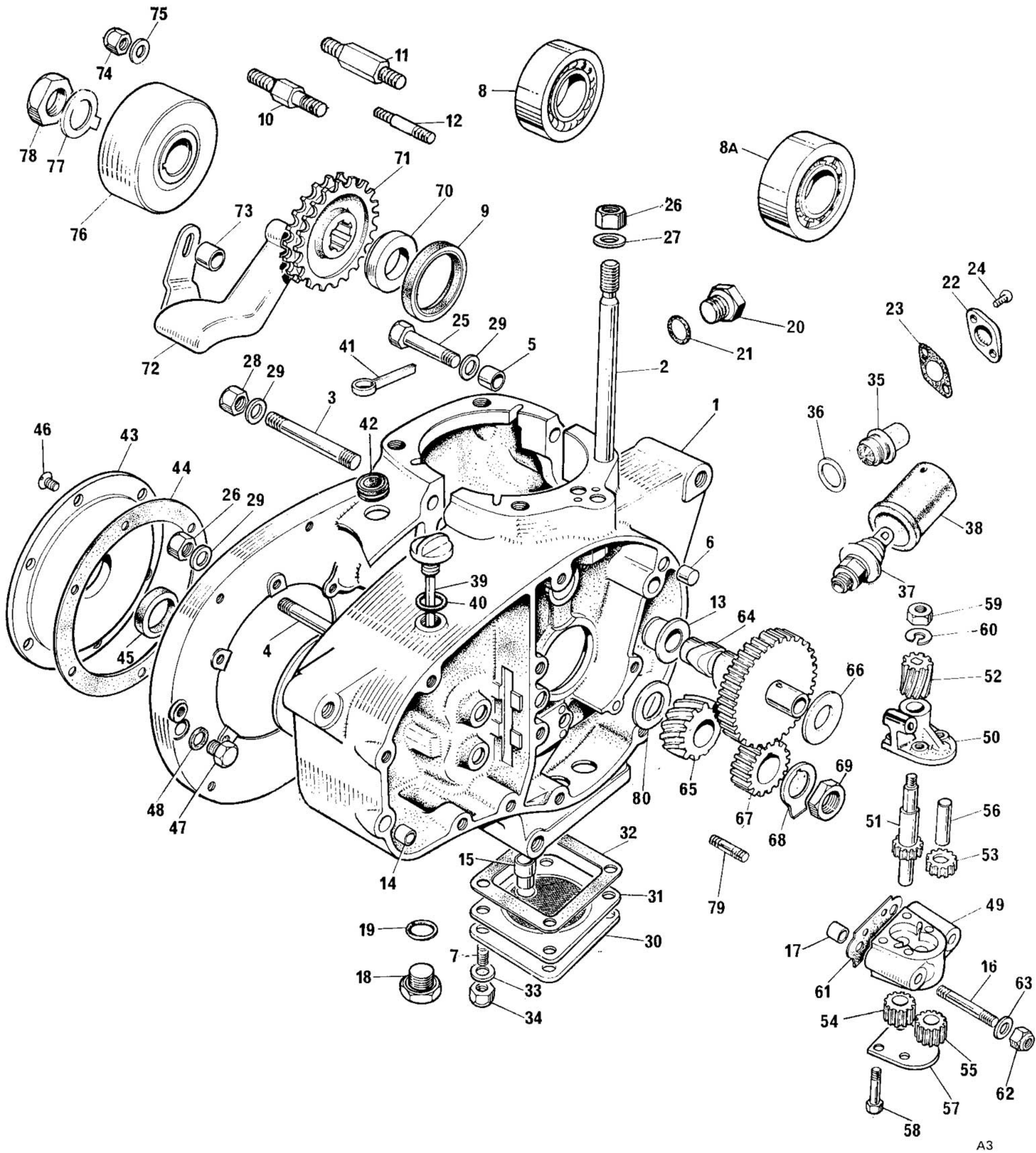
Fig. 3. CRANKCASE
